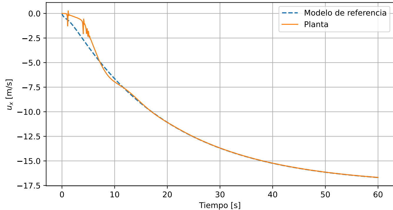
Seguimiento MRAC con paso: u_x
